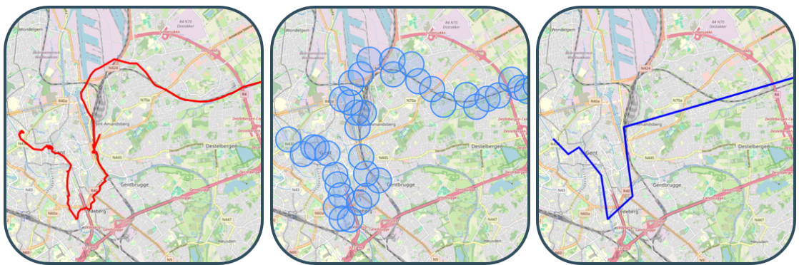
Figure 4.3: Obfuscatiealgoritme gevisualiseerd
