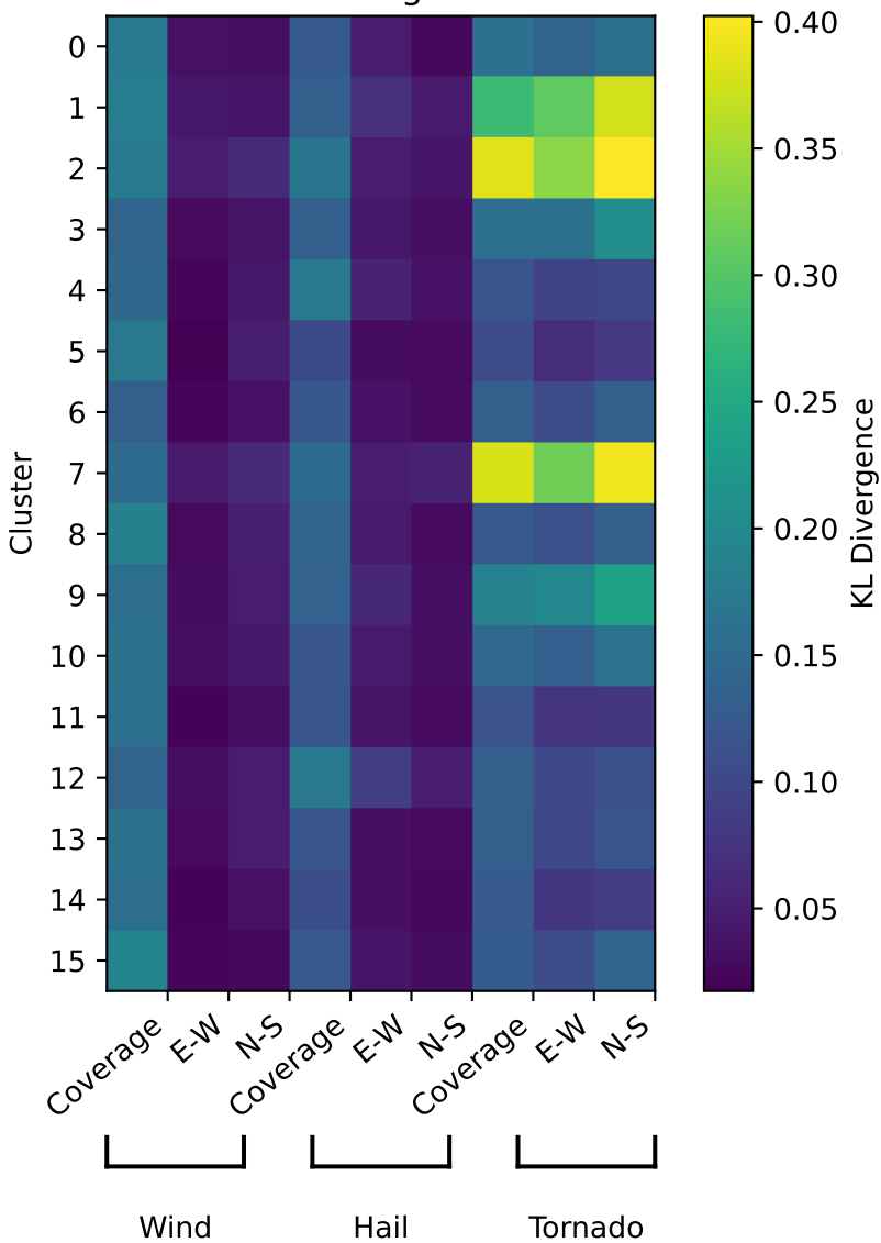
KL Divergence
