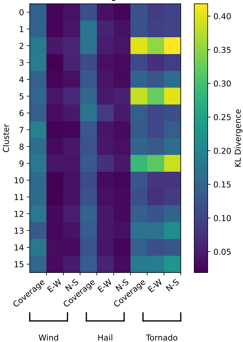
KL Divergence
