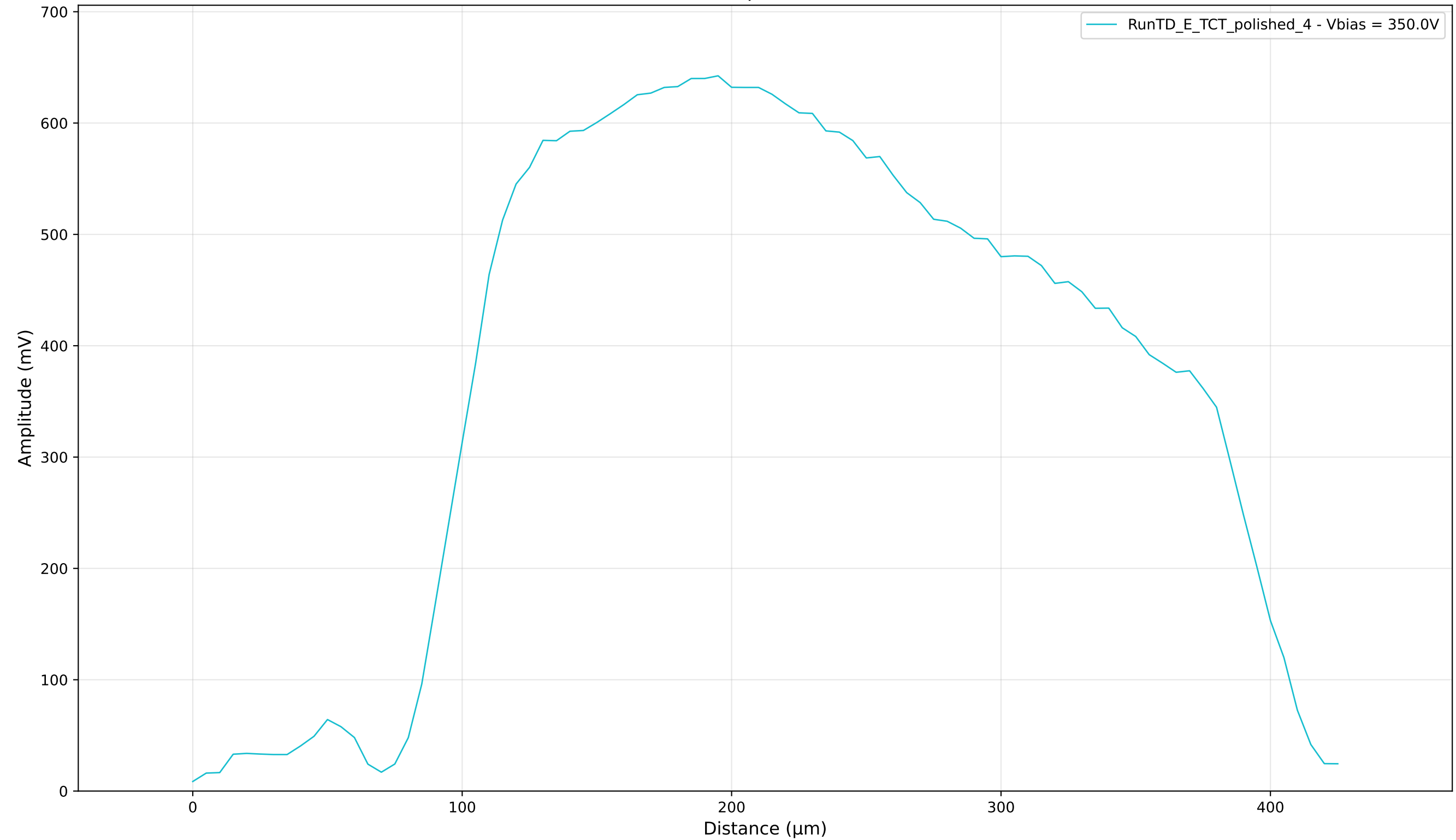
Amplitude
