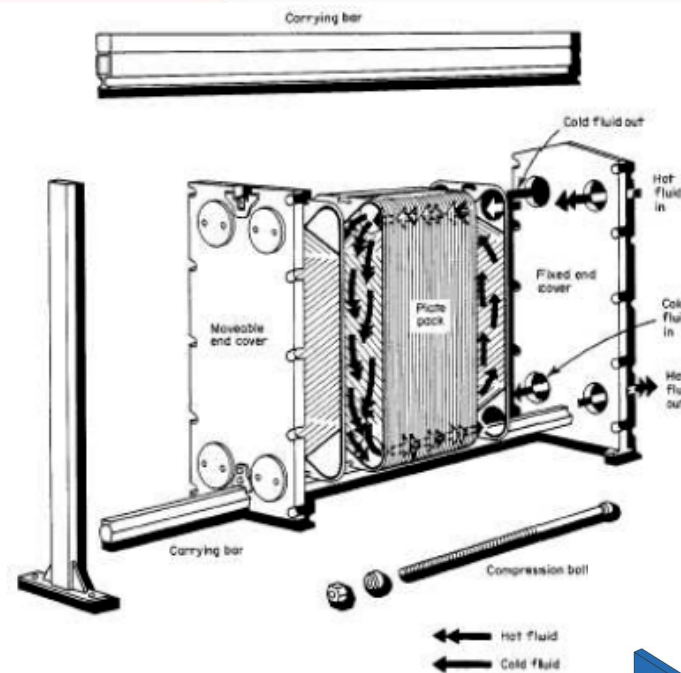
板式換熱器 PHE
