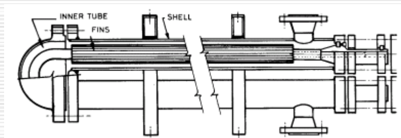
雙套管式換熱器
