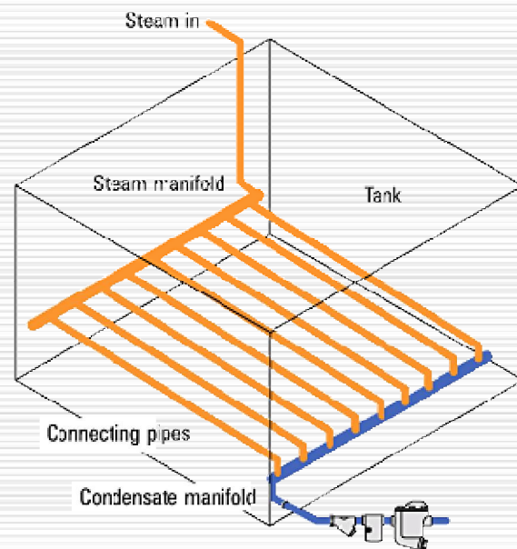
Coil 形換熱器
