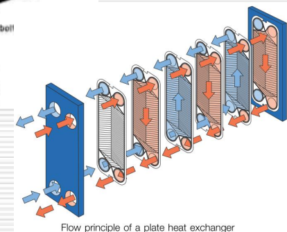
板式換熱器 PHE
