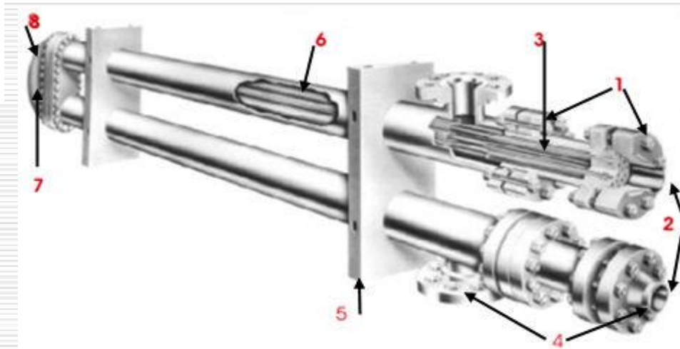
雙套管式換熱器
