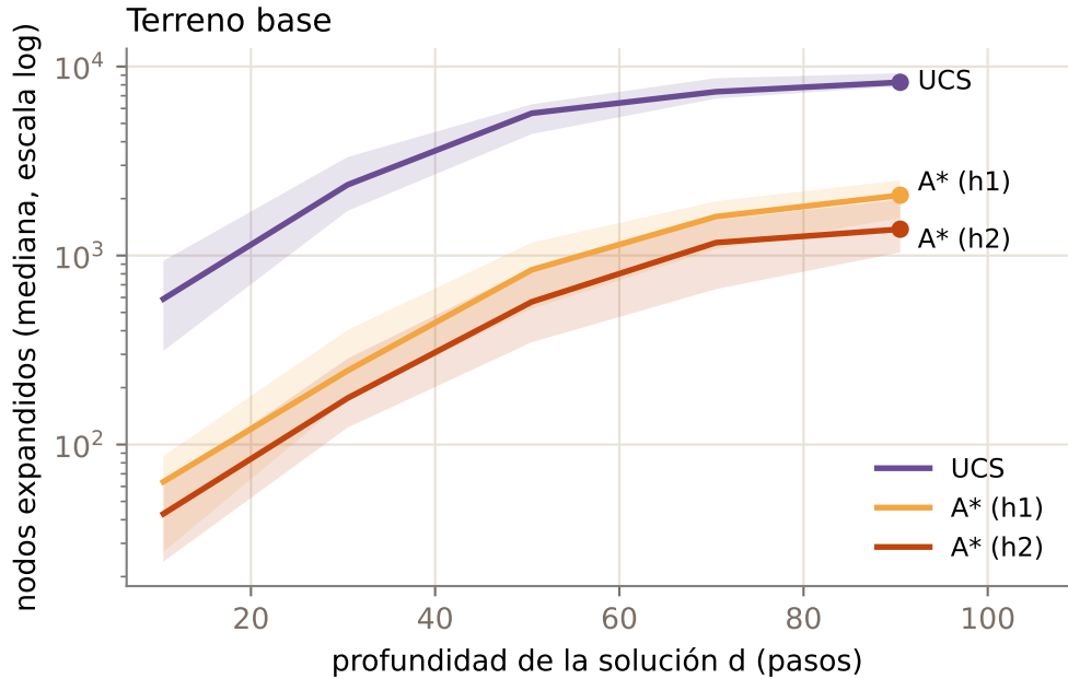
Nodos expandidos frente a la profundidad de la solución (banda: cuartiles 25-75 %)
