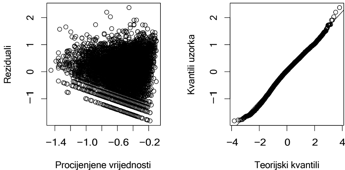
Slika 8: Analiza reziduala: reziduali u ovisnosti o procijenjenim vrijednostima (lijevo) i QQ-plot reziduala (desno)
