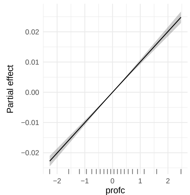
profc
