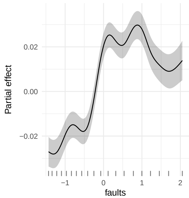
s(faults)
