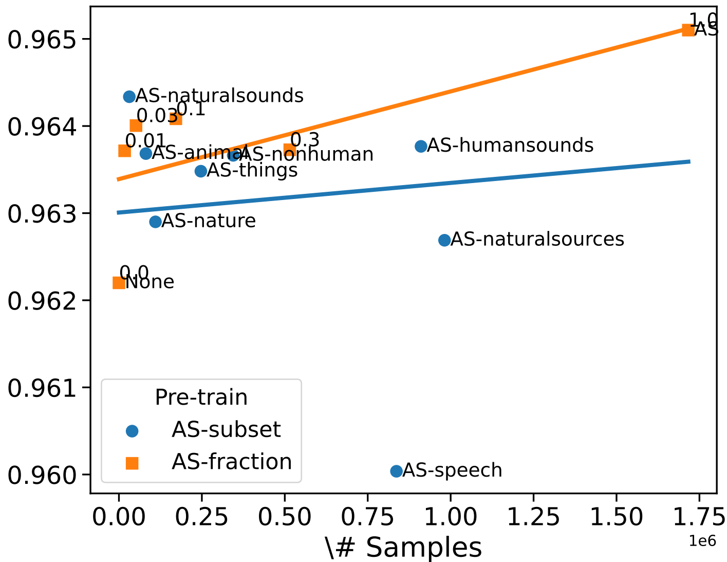
Fine-Tune UAR
