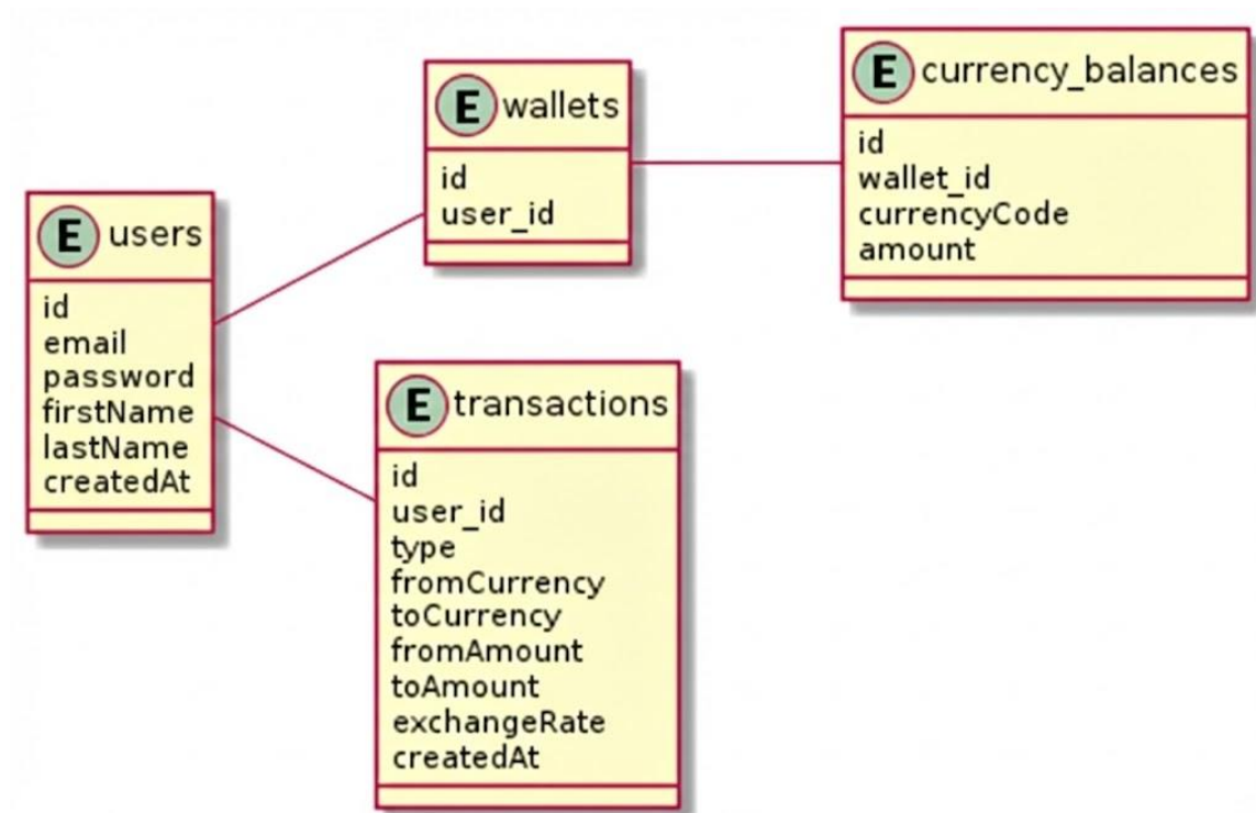
Rysunek 3: Diagram ERD
