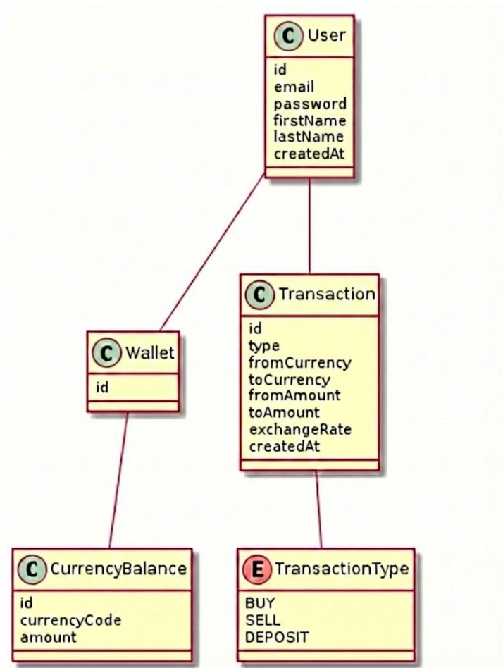
Rysunek 2: Diagram klas
