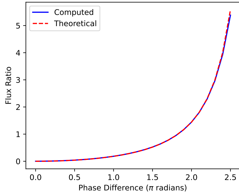
Sidelobe/Centre Flux
