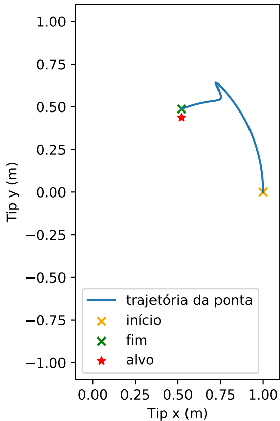
Trajetória da ponta - PIRL (PI-reward), seed=4, high_energy_success
