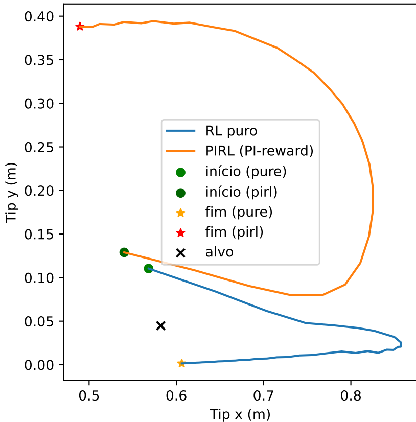
Trajetória da ponta - seed=0, high_energy_success
