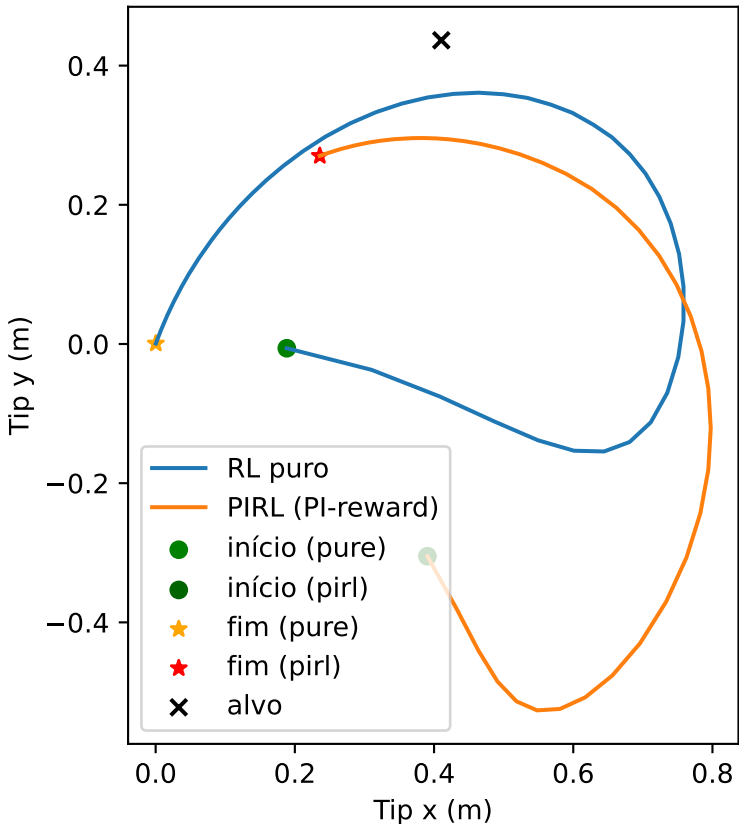
Trajectoria da ponta - seed=3, high_energy_fail
