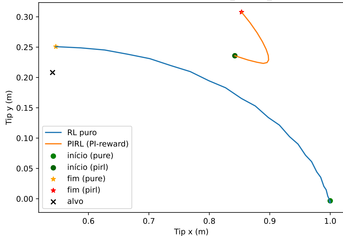
Trajetória da ponta - seed=3, low_energy_success
