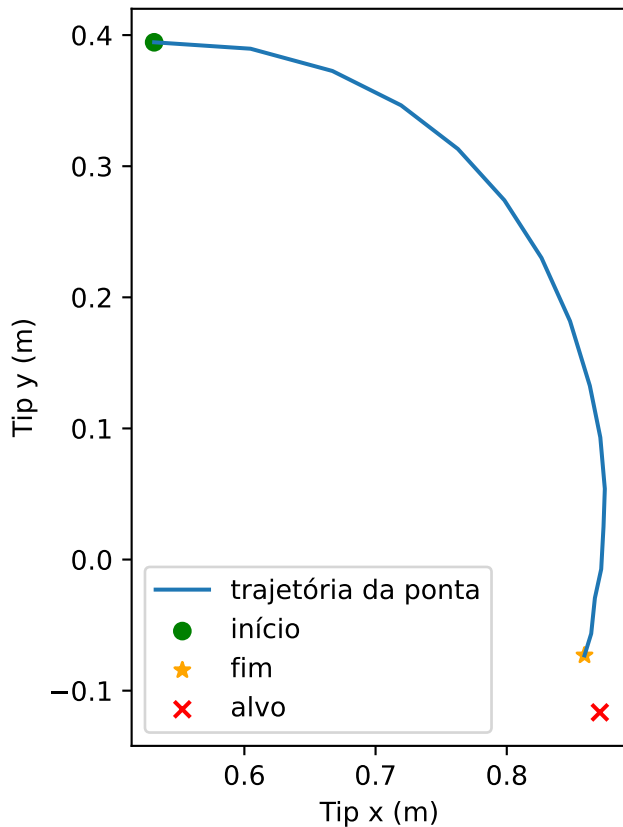
Trajeto ria da ponta - PIRL (PI-reward), seed=0, low_energy_success
