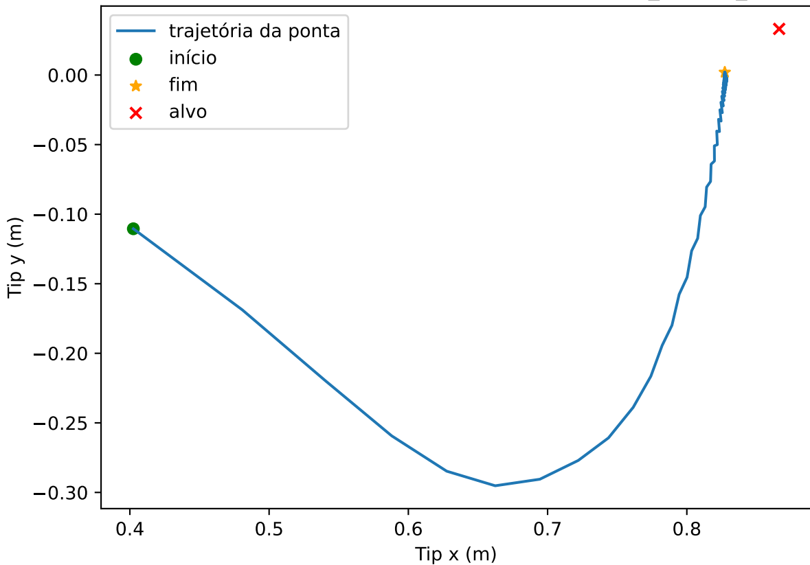
Trajetória da ponta - PIRL (PI-reward), seed=1, high_energy_success
