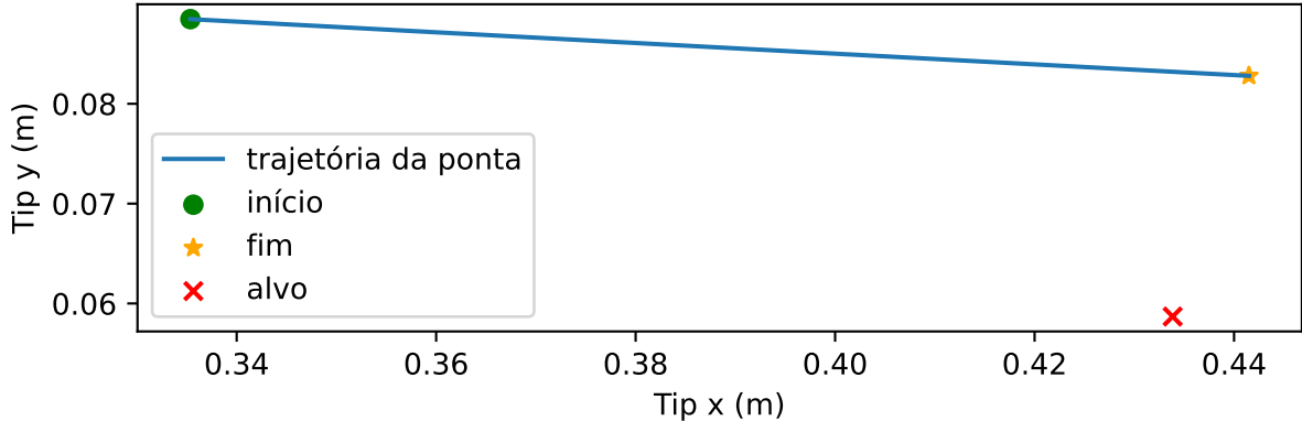
Trajetória da ponta - PIRL (PI-reward), seed=1, low_energy_success
