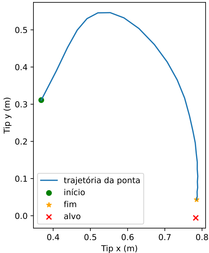
Trajetória da ponta - PIRL (PI-reward), seed=2, high_energy_success
