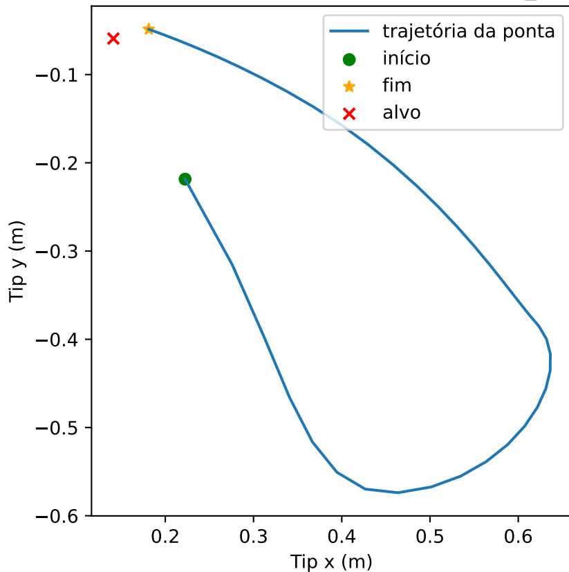
Trajetória da ponta - PIRL (PI-reward), seed=3, high_energy_success
