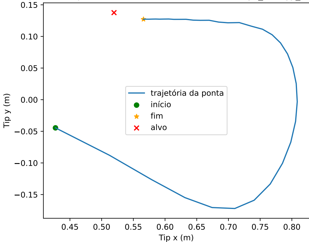
Trajetória da ponta - PIRL (PI-reward), seed=4, high_energy_success
