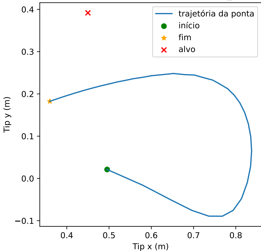
Trajetória da ponta - RL puro, seed=0, high_energy_fail
