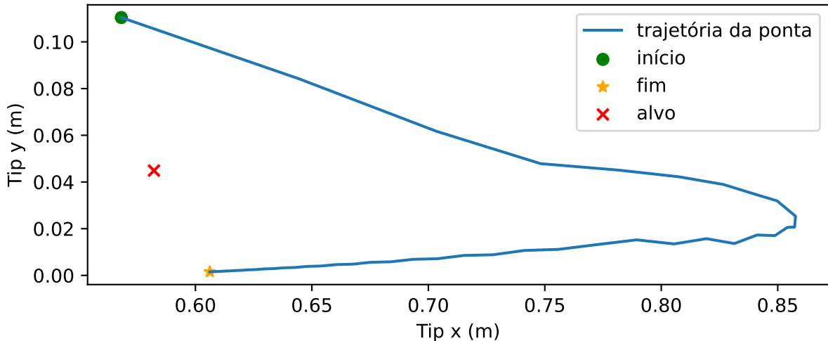
Trajetória da ponta - RL puro, seed=0, high_energy_success
