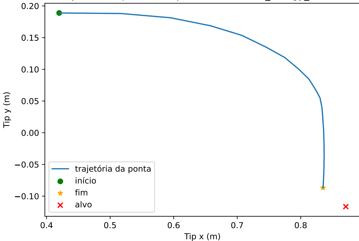
Trajetória da ponta - RL puro, seed=0, low_energy_success
