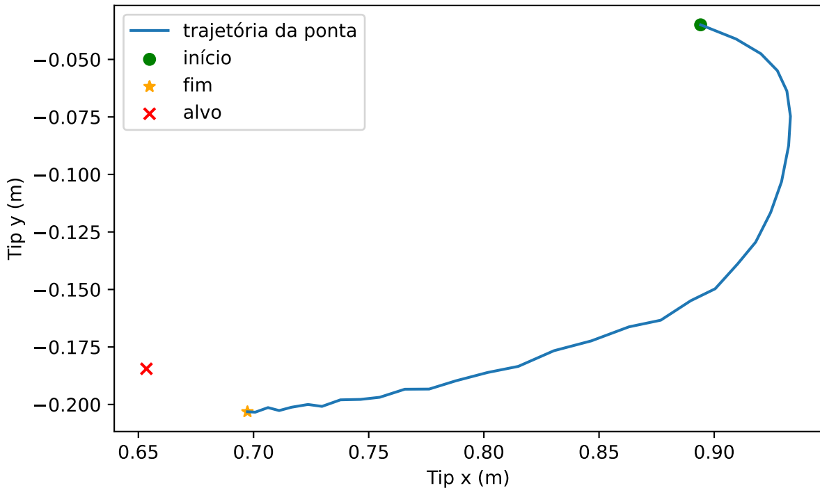
Trajetória da ponta - RL puro, seed=1, low_energy_success
