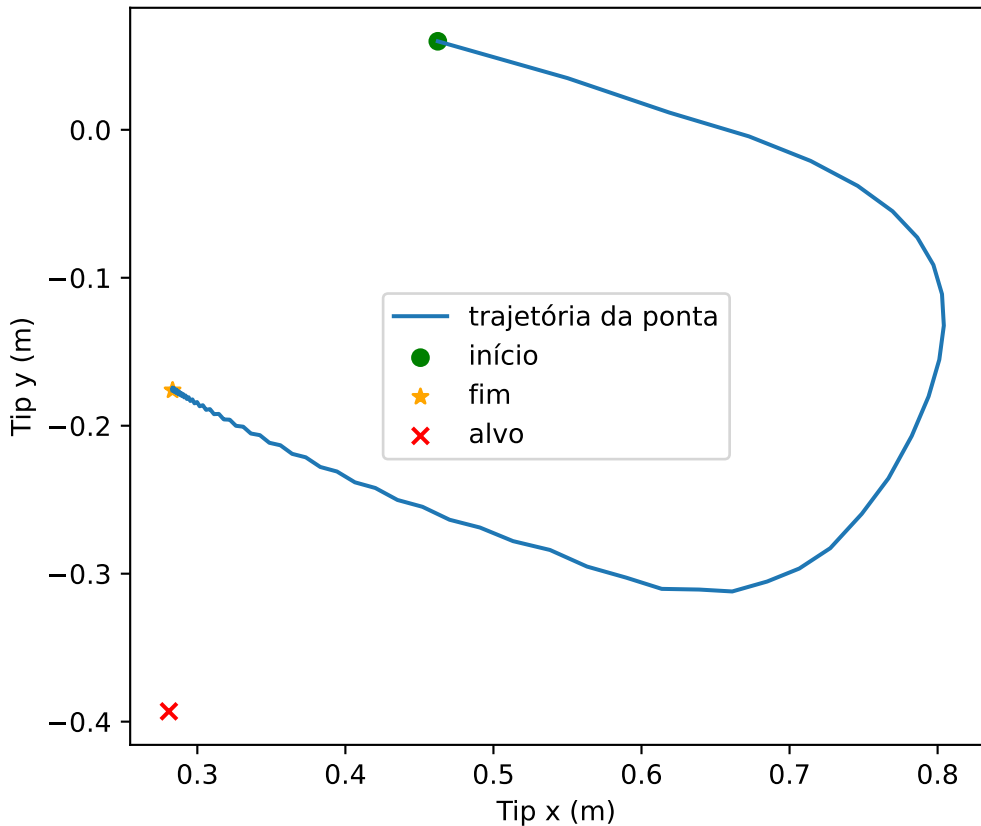
Trajetória da ponta - RL puro, seed=2, high_energy_fail
