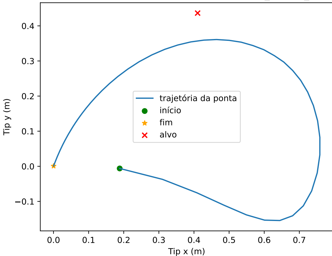
Trajetória da ponta - RL puro, seed=3, high_energy_fail
