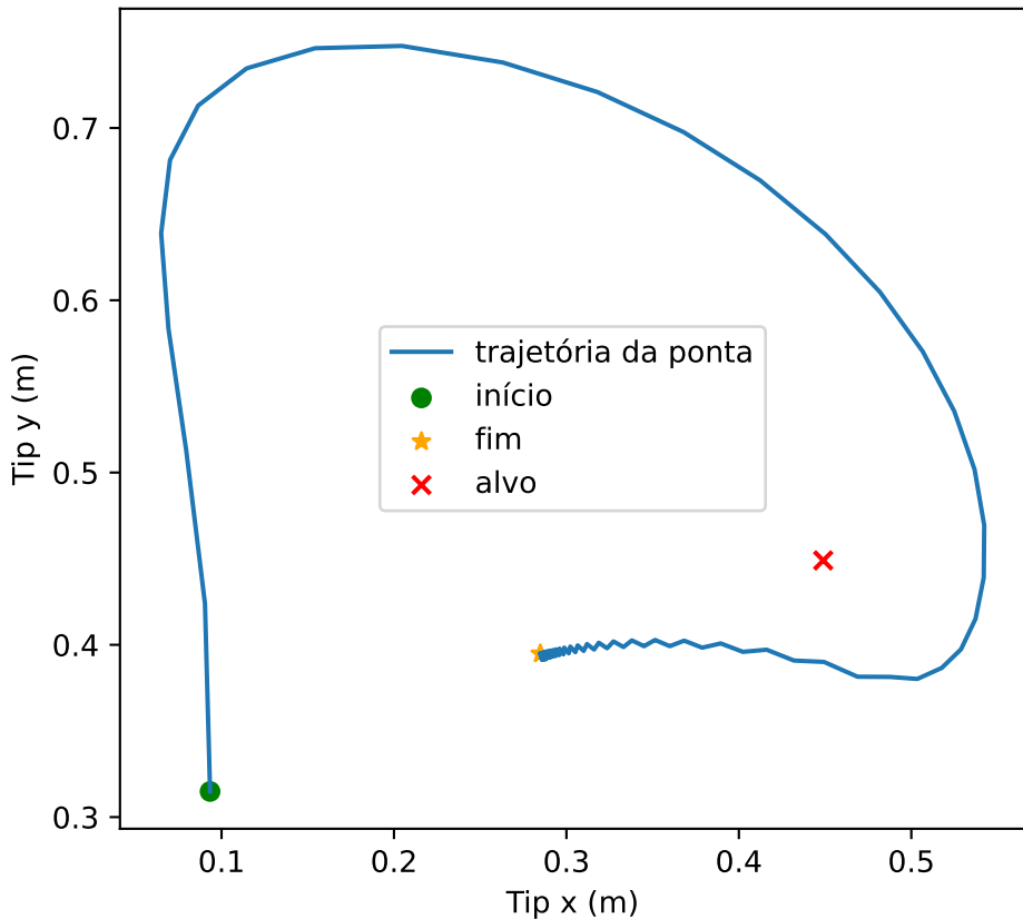
Trajeto ria da ponta - RL puro, seed=4, high_energy_fail
