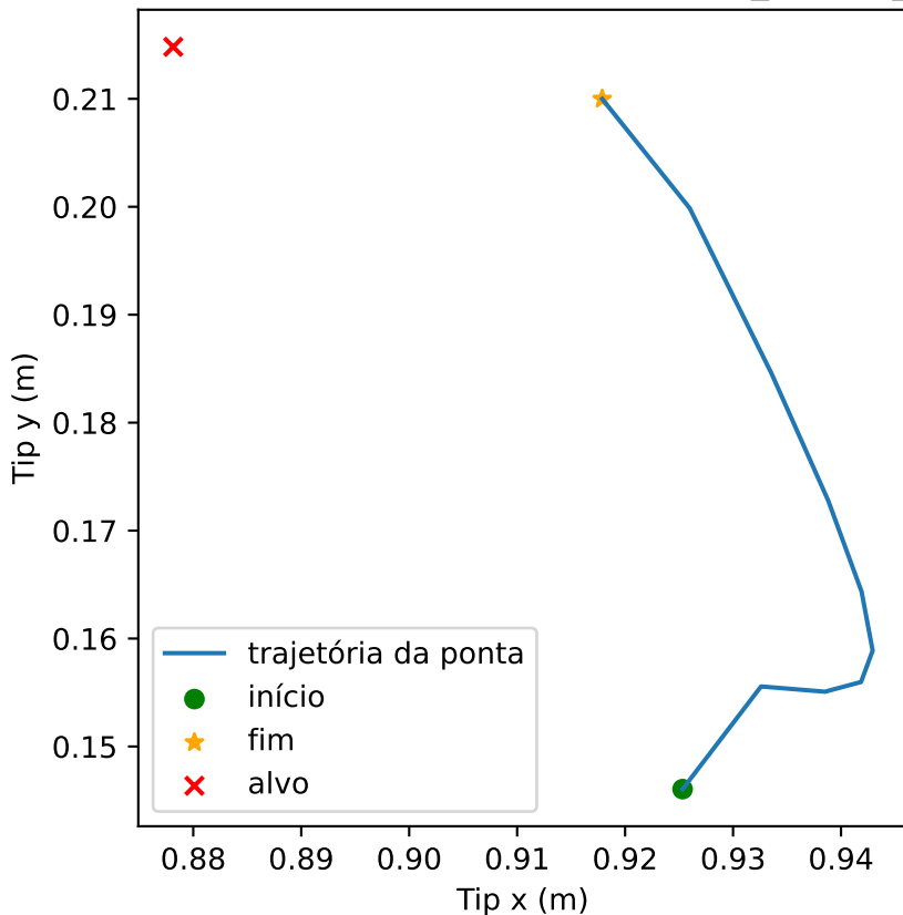
Trajetória da ponta - RL puro, seed=4, low_energy_success
