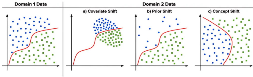
Σχήμα 2.19: Είδη μετατόπισης τομέα. (Ganin et al. 2016)
