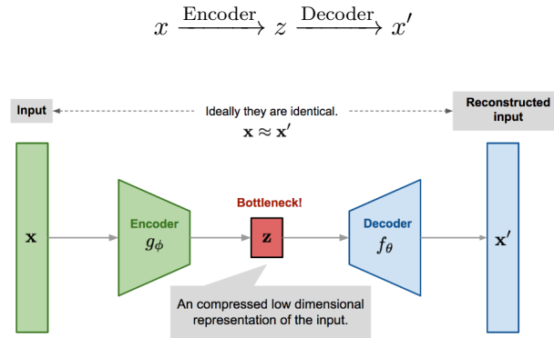
Σχήμα 3.26: Αρχιτεκτονική ενός Autoencoder. (Akkus et al. 2023)
