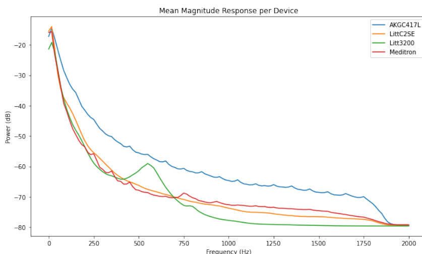
Σχήμα 2.12: Απεικόνιση της μέσης απόκρισης συχνότητας των διαφορετικών συσκευών καταγραφής.
