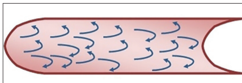
Σχήμα 2.3: Τυρβώδης ροή αέρα. (Sarkar et al. 2015)
