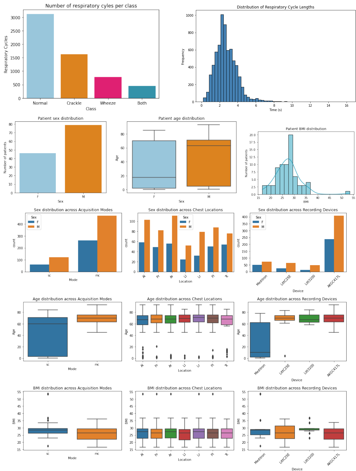
Σχήμα 2.11: Σύντομη στατιστική περιγραφή της βάσης δεδομένων RSDB.
