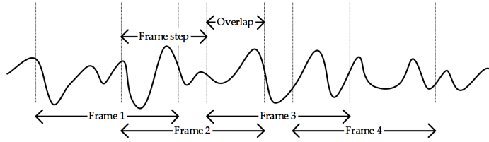
Σχήμα 2.15: Τεμαχισμός σήματος σε frames με επικάλυψη. (Διαδίκτυο)
