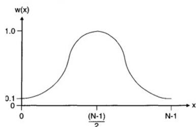
Σχήμα 2.17: Παράθυρο Hamming. (Διαδίκτυο)
