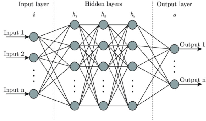
Σχήμα 3.25: Αρχιτεκτονική ενός MLP.
