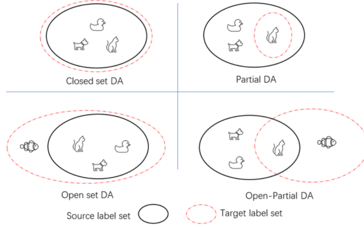
Σχήμα 2.21: Κατηγορίες προσαρμογής τομέα. (Fan et al. 2022)
