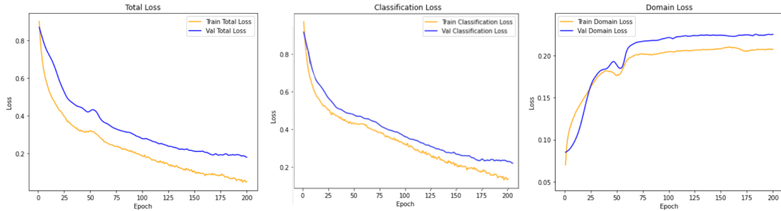
Σχήμα 4.14: Συναρτήσεις κόστους του CDAN.
