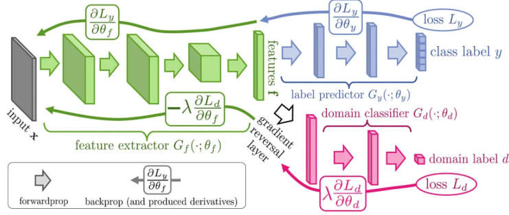
Σχήμα 3.27: Αρχιτεκτονική ενός DANN. (R. Wang et al. 2019)
