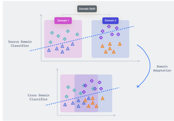
Σχήμα 2.18: Βασική αρχή λειτουργίας της προσαρμογής πεδίου. (Kundu 2022)
