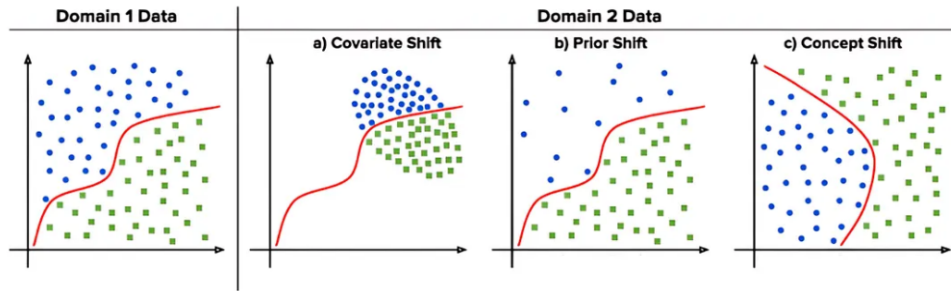
Σχήμα 2.17: Είδη μετατόπισης πεδίου. (Ganin et al. 2016)
