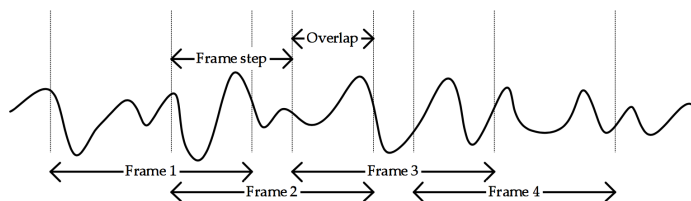
Σχήμα 2.14: Τεμαχισμός σήματος σε frames με επικάλυψη. (Διαδίκτυο)
