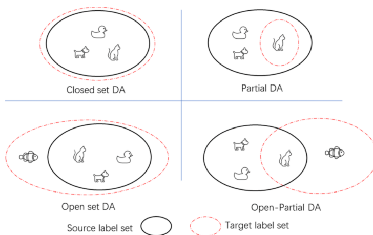
Σχήμα 2.19: Είδη προσαρμογής πεδίου. (Fan et al. 2022)
