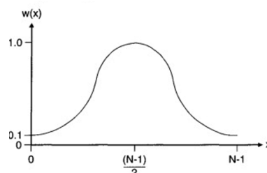
Σχήμα 2.15: Παράθυρα Hann και Hamming. (Διαδίκτυο)
