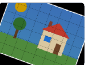
rotate 20°
