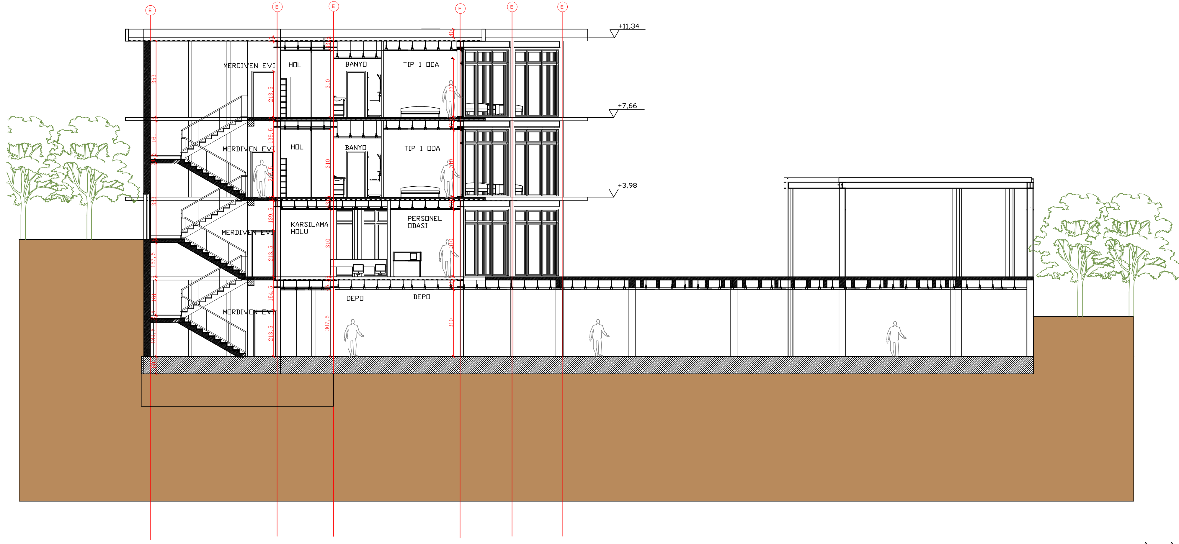
A-A KESİT
