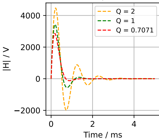
Bandpass
