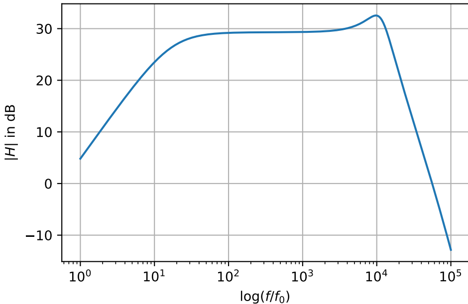
Betragsfrequenzgang
