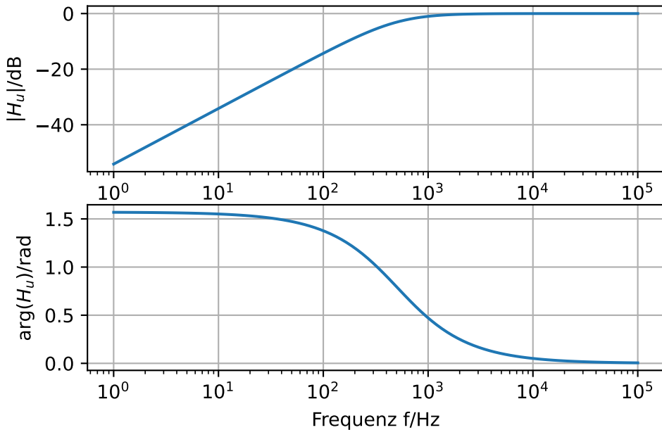
Bode-Diagramm einer RC-Schaltung
