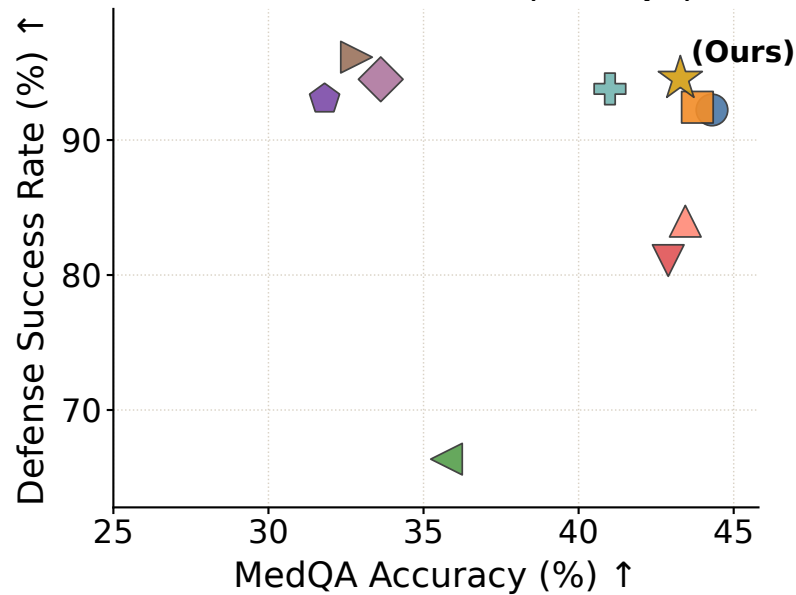
Llama-2-7B-Chat (MedQA)
