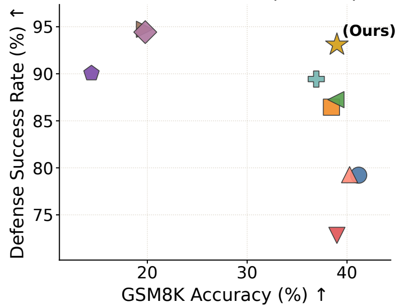
Llama-2-7B-Chat (GSM8K)
