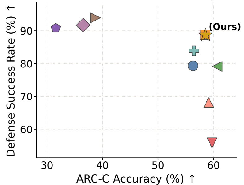
Llama-2-7B-Chat (ARC-C)
