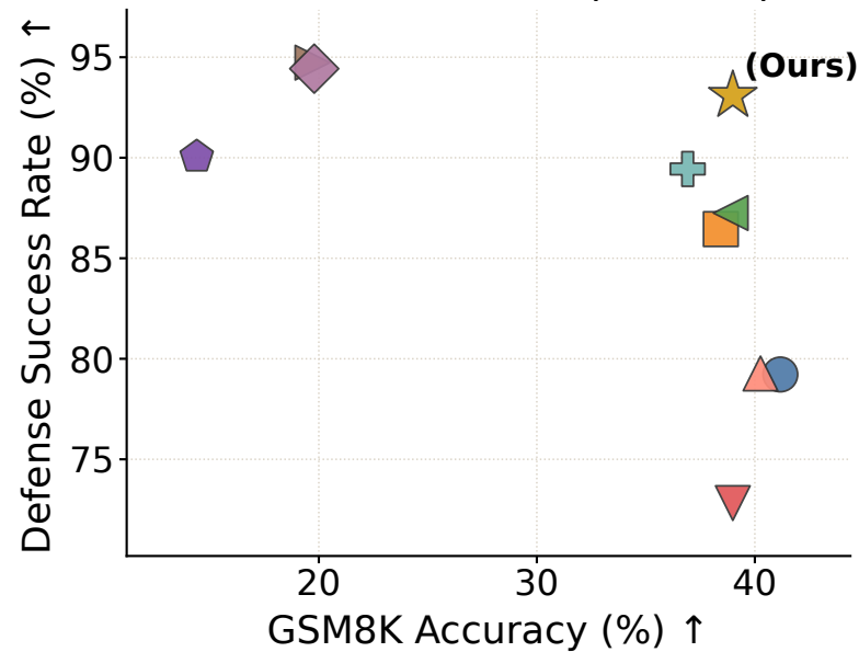
Llama-2-7B-Chat (GSM8K)
