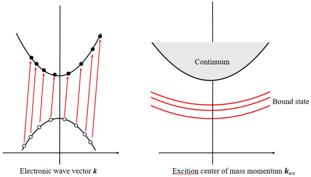
圖 2.3：單粒子載子對之集體相干疊加與雙粒子激子本徵色散能譜示意圖。(左) 在單粒子電子波向量 \mathbf{k} 空間中，價帶電洞 (空心圓) 與導帶電子 (實心圓) 受特定質心動量 \hbar\mathbf{k}_{\text{ex}} 聯結的集體多體躍遷 (紅色箭頭)；(右) 經由求解 Bethe-Salpeter 方程式對角化後，於激子質心動量 k_{\text{ex}} 空間中，在準粒子連續帶 (Continuum) 下方所凝聚出的離散激子束縛態 (Bound state) 本徵色散能帶 (紅線)。
