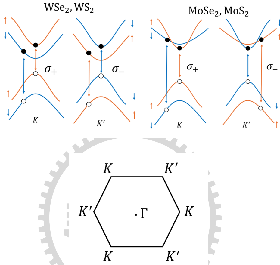
圖 1.3：單層過渡金屬二硫族化合物（TMD）之谷能帶結構與布里淵區示意圖。上方左側為鎢系材料（WSe 2 , WS 2 ）與右側為鉬系材料（MoSe 2 , MoS 2 ）於 K 與 K' 谷之能帶自旋分裂及光學選擇定則；下方為對應之六方第一布里淵區幾何示意圖。
