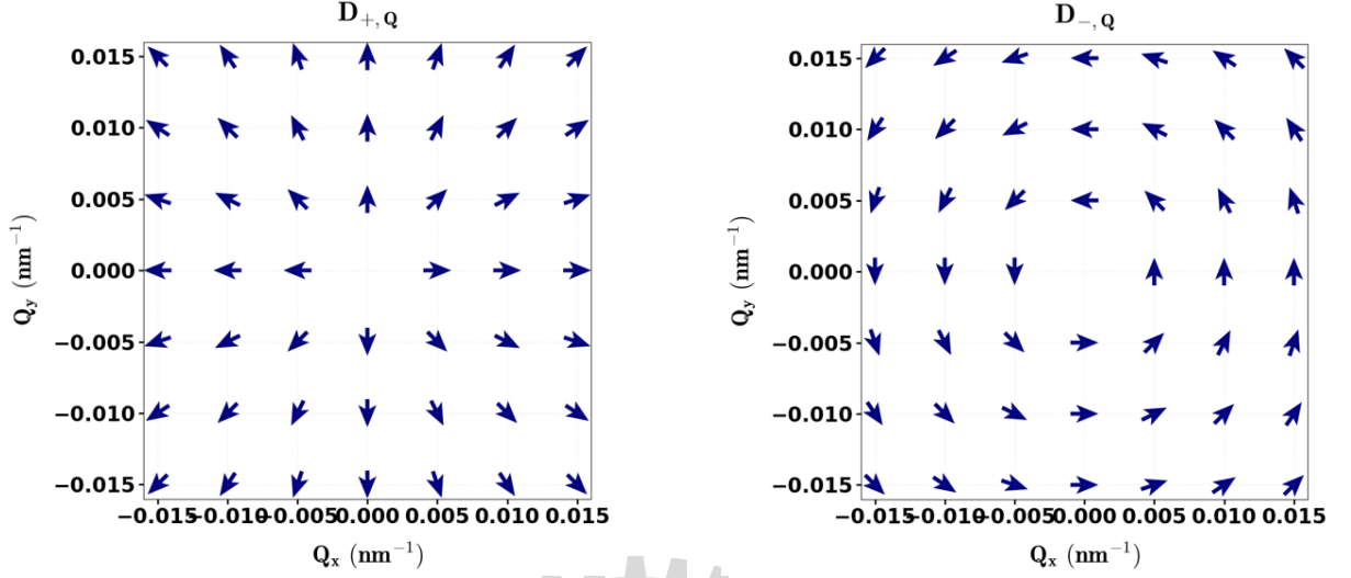
(a) 縱向類光上能帶 D_{+,Q} ：偶極矩方向平行於質心動量 \mathbf{Q} ，呈輻射狀分佈。
