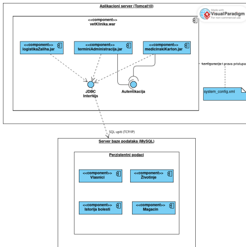
Slika: Dijagram komponenti
