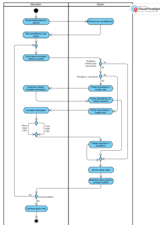
Slika: Dijagram aktivnosti
