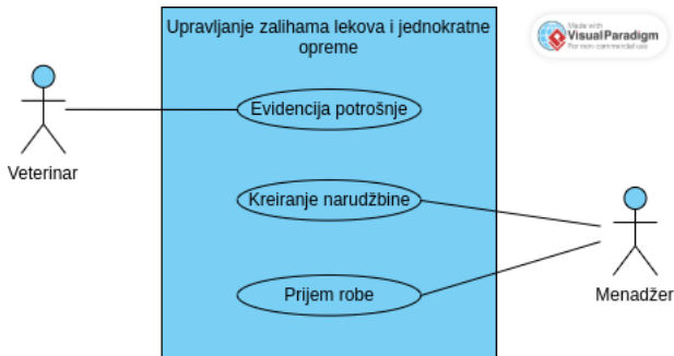
Slika: Dijagram slučaja upotrebe
