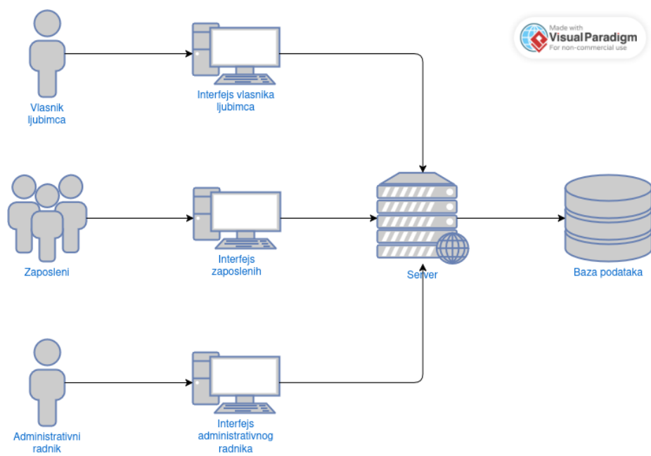
Slika 1: Dijagram arhitekture
