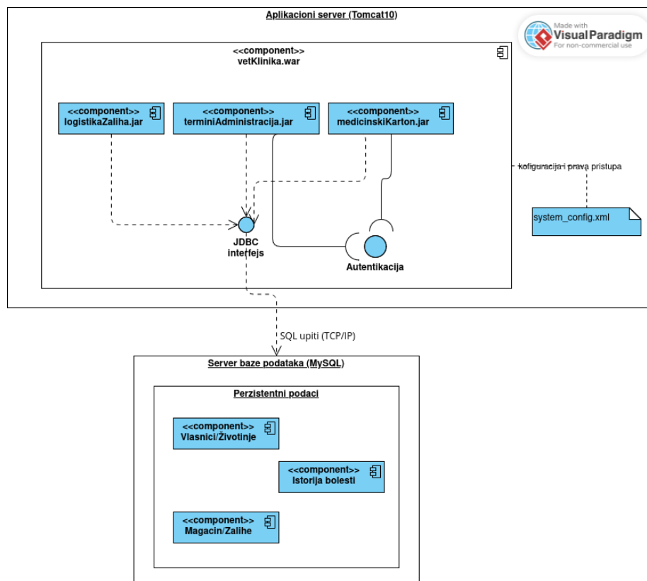
Slika 2: Dijagram komponenti
