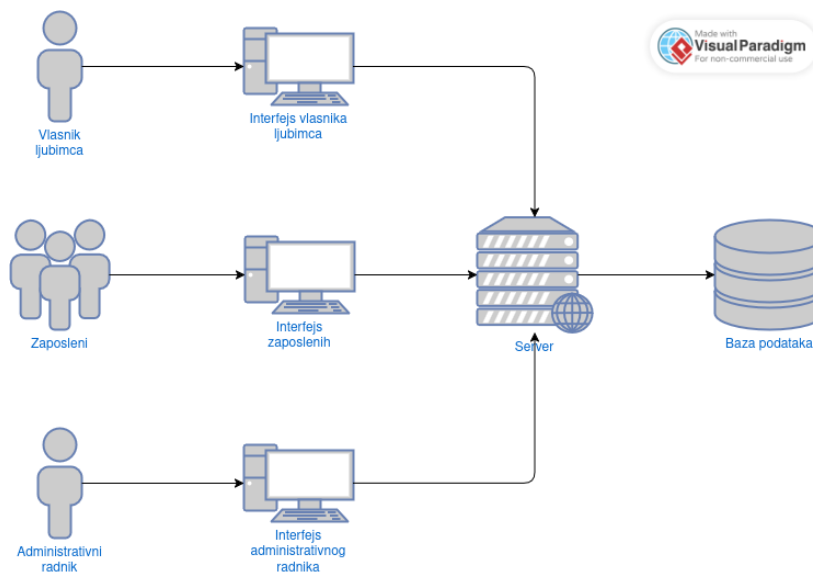
Slika 16: Dijagram arhitekture
