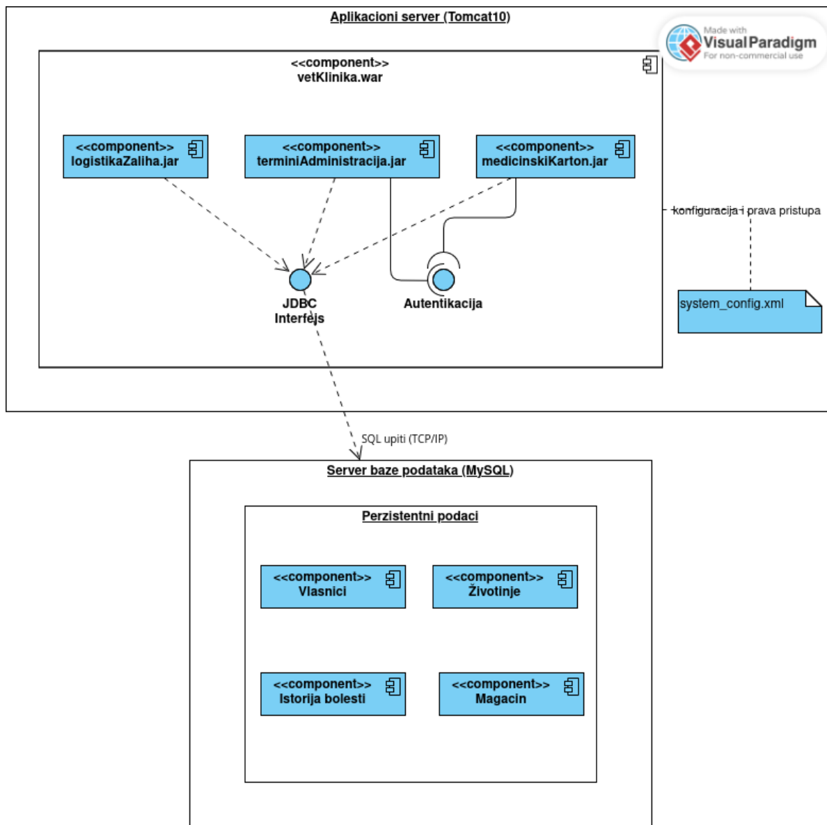
Slika 17: Dijagram komponenti
