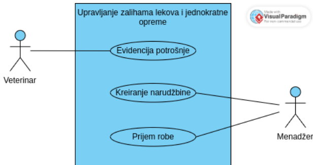
Figure: Dijagram slučaja upotrebe
