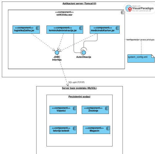
Figure: Diagram komponenti
