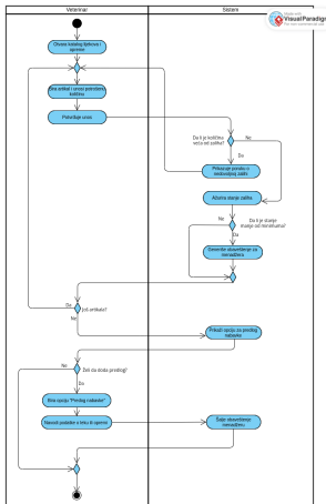
Figure: Dijagram aktivnosti
