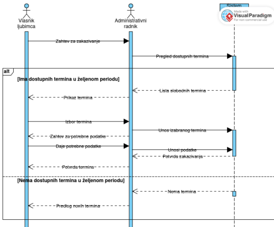
Figure: Dijagram sekvence
