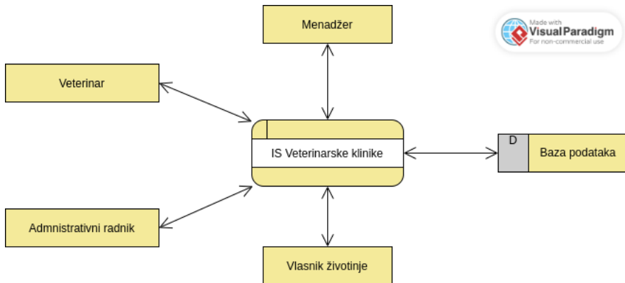
Figure: Dijagram konteksta
