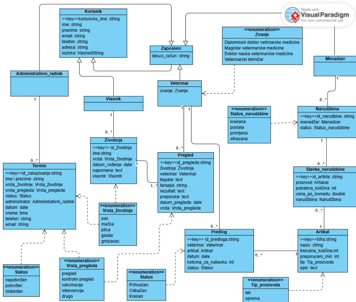
Slika 17: Dijagram klasa podataka
