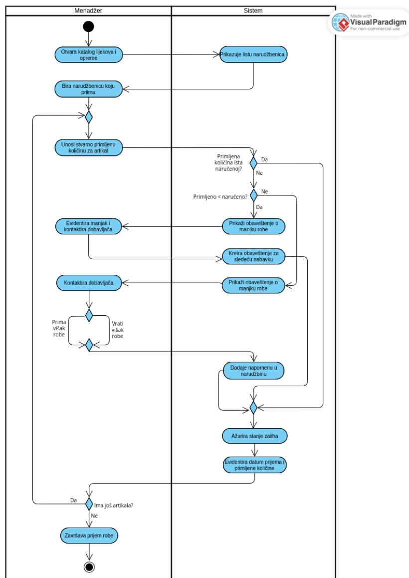
Slika 16: Dijagram aktivnosti - Prijem robe
