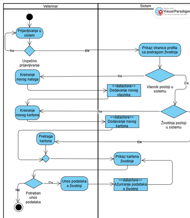
Slika 11: Dijagram aktivnosti: Unos podataka o životinji
