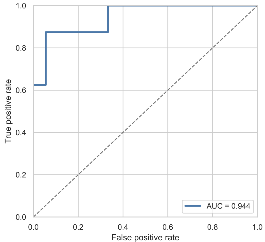
B. ROC curve (n=26)
