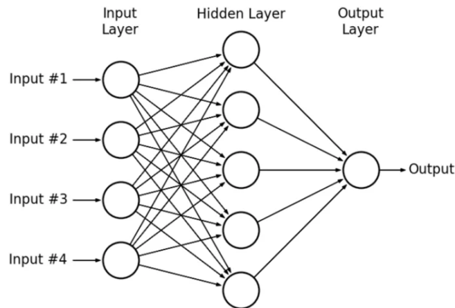
Figura 2.3: Una rete feedforward con un input layer a 4 nodi, un hidden layer a 5 nodi e un output layer a un nodo: ogni connessione porta con sé un peso appreso, omissso per chiarezza.
