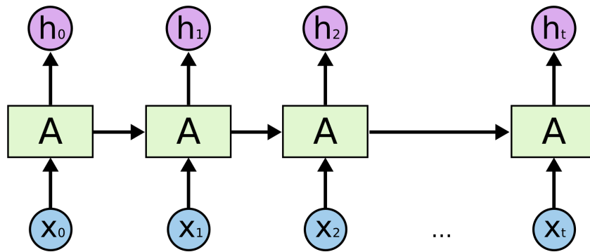
Figura 2.6: La rete ricorrente srotolata lungo il tempo: il modulo A rappresenta la funzione ricorrente, ad esempio l'Equazione 2.4, riapplicata con gli stessi pesi a ogni istante.
