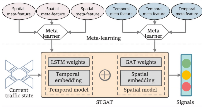
Figura 3.2: Principio del meta-apprendimento applicato da MetaSTGAT: le meta-feature spaziali e temporali condizionano, tramite un meta-learner dedicato, i pesi dei layer LSTM e GAT usati per elaborare lo stato corrente del traffico. Adattato da Wang et al. (2022).
