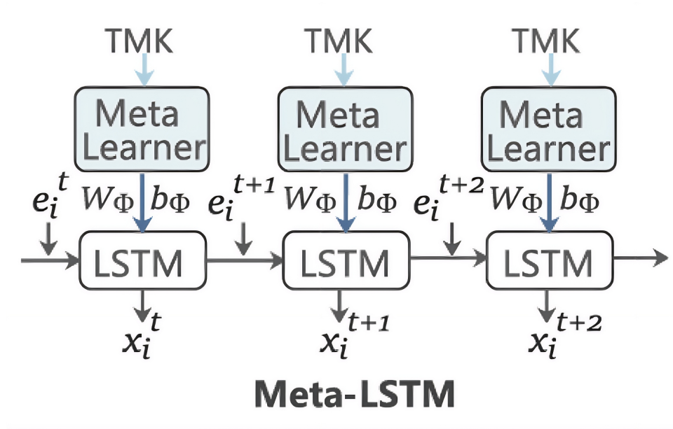
Figura 3.5: Meta-LSTM "srotolata" nel tempo: a ogni istante t il meta-learner genera, da \text{TMK}(i) , i pesi W_\Phi e b_\Phi della cella LSTM che produce x_i^t dall'input e_i^t e dallo stato nascosto precedente h_i^{t-1}, c_i^{t-1} . Adattato da Wang et al. (2022).
