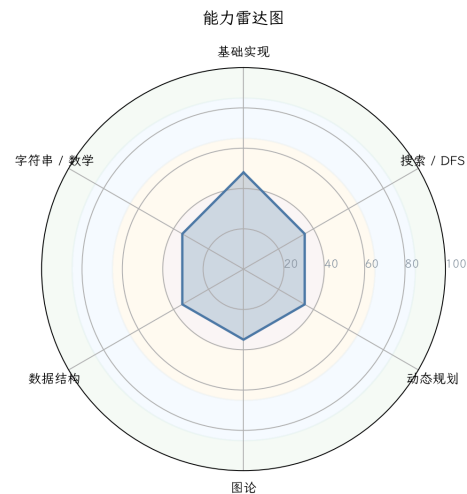
图 1：能力雷达图
