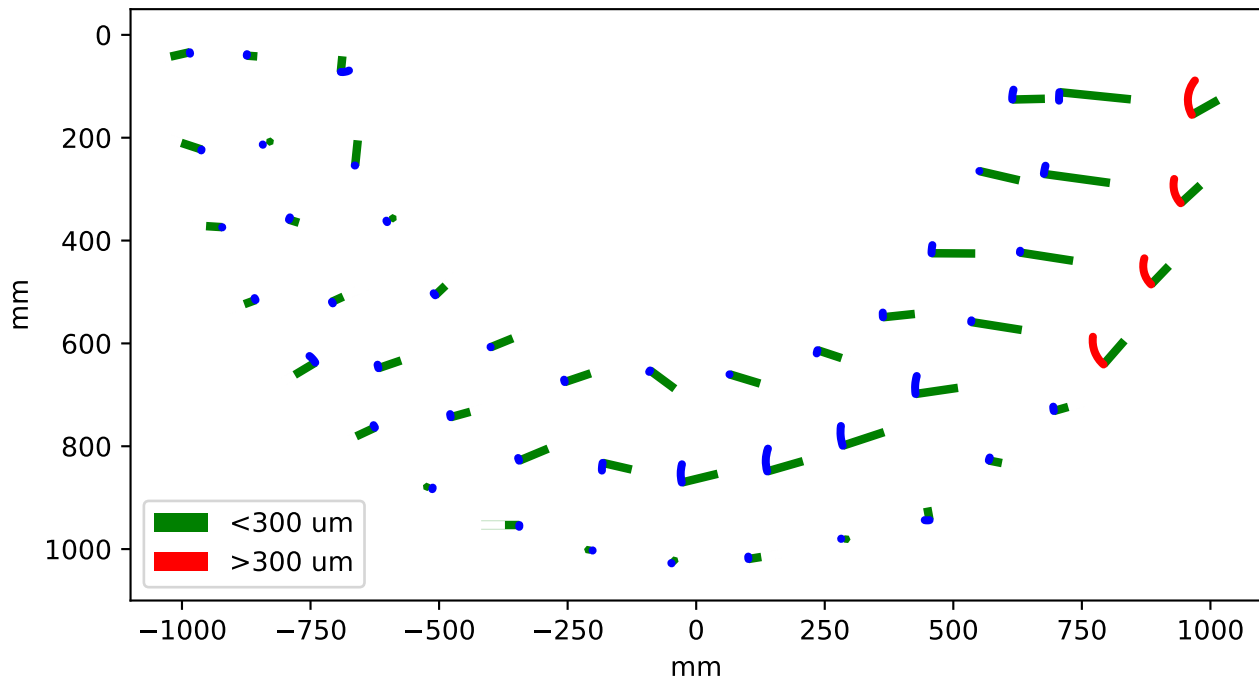
DD12-O-103, Module positions, Bottom side
