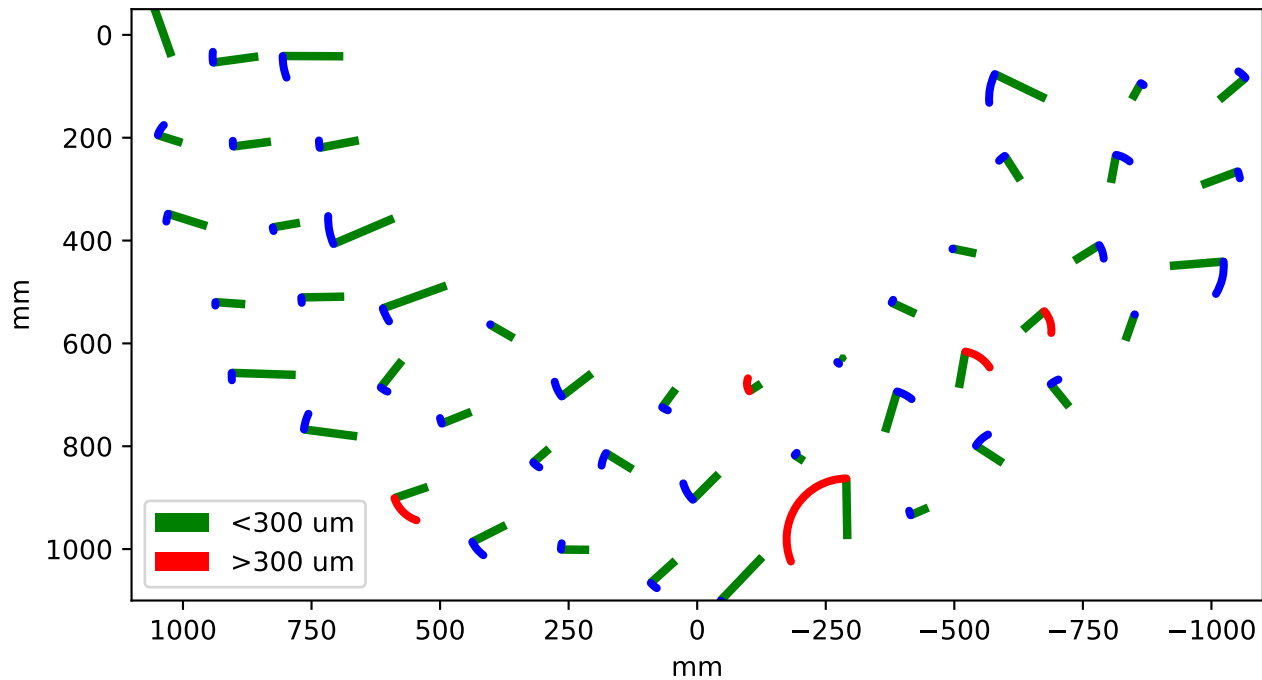
DD12-O-103, Module positions, Top side
